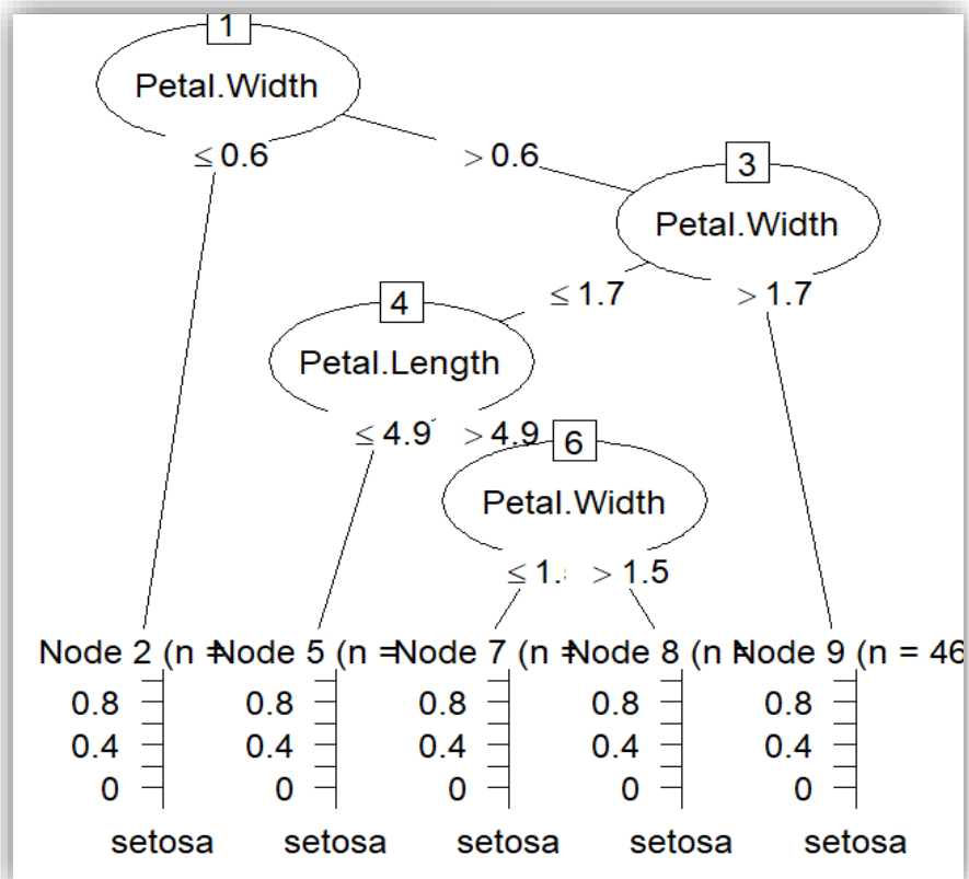
Figura 1. Árbol de decisión generado mediante J48 en RStudio utilizando el conjunto de datos Iris.
